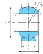
GEG...ET-2RS
