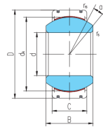
GEG...XT-2RS
